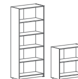
SR-5W 770 x 359 x 1815 SR-2W 770 x 359 x 790
