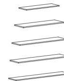
B 840 1376 x 450 x 25 B 830 1426 x 450 x 25 B 860 1801 x 450 x 25 B 850 1851 x 450 x 25 B 870 2276 x 450 x 25
