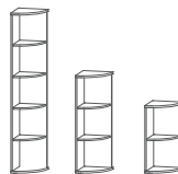
УС-1 365 x 365 x 823 УС-2 365 x 365 x 1200 УС-3 365 x 365 x 1975
