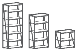
LMHC 80 800 x 430 x 2253 LMMC 80 800 x 430 x 1517 LMLC 80 800 x 430 x 781
